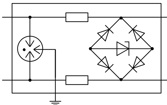
Рис. 18 УЗИП с мостовой схемой
