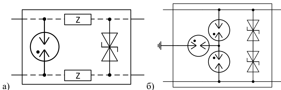
Рис. 15 Многоступенчатое УЗИП а) с согласующими элементами, включёнными в защищаемую линию; б) без согласующих элементов
