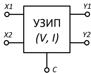
г) – пятивыводное УЗИП
